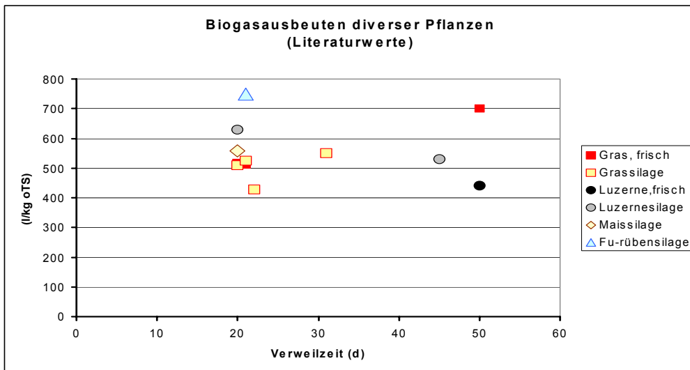
Abbildung 2: Biogasausbeuten aus Pflanzen (Laborversuche)
